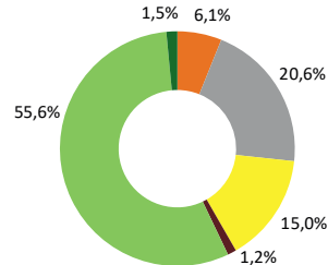
Verbleibender Energieträgermix
